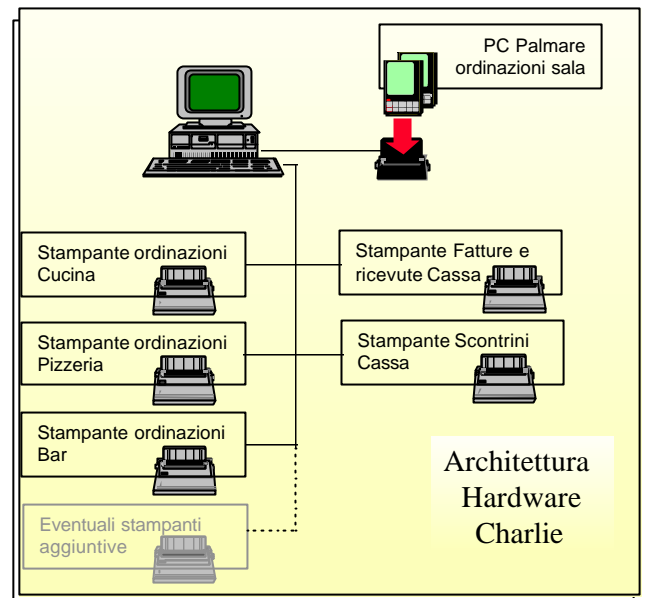
Schema con trasmissione via Cavo
